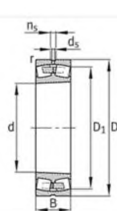
圆锥孔 K = 锥度 1 : 12、 K30 = 锥度 1 : 30
