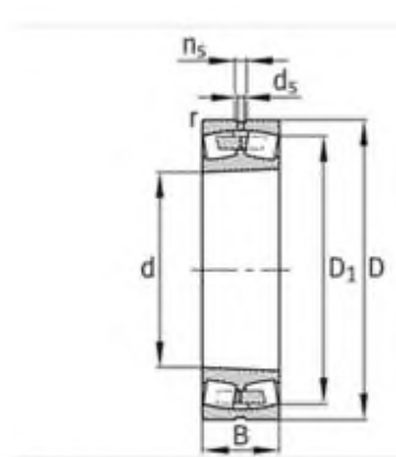
圆锥孔 K = 锥度 1 : 12、 K30 = 锥度 1 : 30
