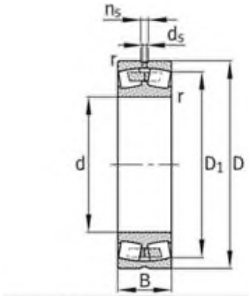
带中挡边 圆柱孔
