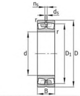
带中挡边 圆柱孔
