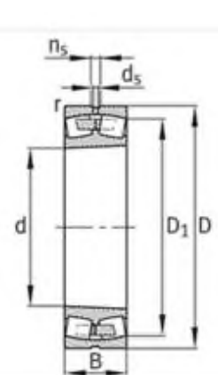
圆锥孔 K = 锥度 1 : 12、 K30 = 锥度 1 : 30
