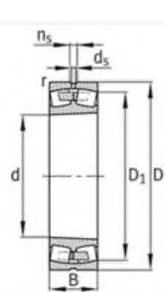
圆锥孔 K = 锥度 1 : 12、 K30 = 锥度 1 : 30
