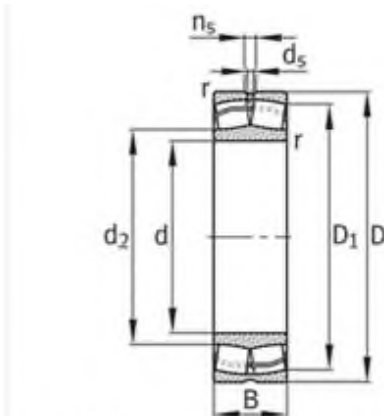
E1 设计 圆柱孔
