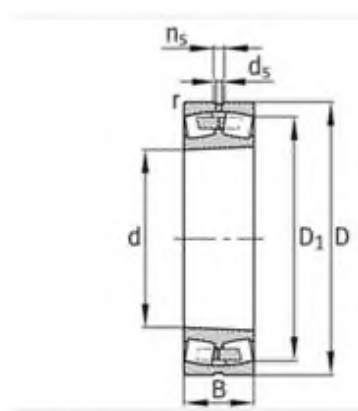
圆锥孔 K = 锥度 1 : 12、 K30 = 锥度 1 : 30
