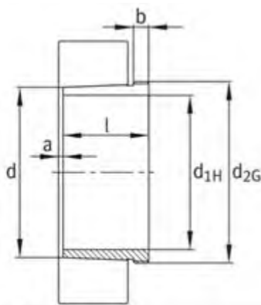
锥度为 1 : 12
