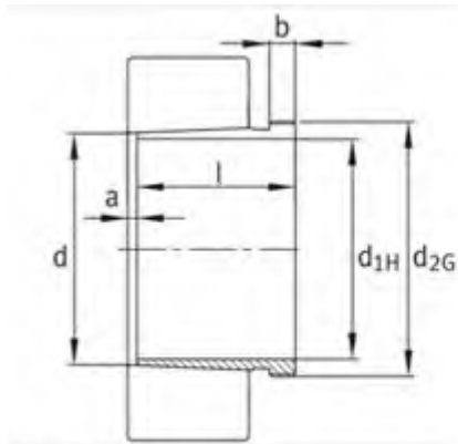
AH240、AH241 锥度为 1 : 30
