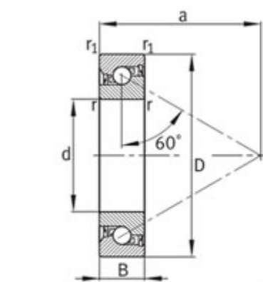
7602..-2RS、 7603..-2RS、 BSB..-2RS
